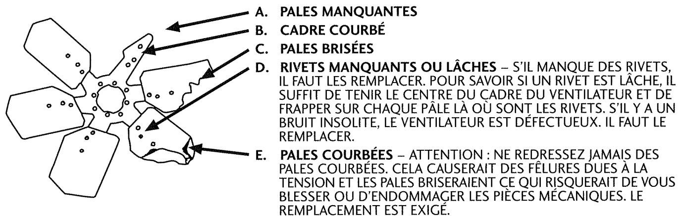
FIG. #1 IMPORTANT – REMPLACEZ TOUJOURS LES VENTILATEURS ENDOMMAGÉS Points à surveiller lors de l’inspection de l’embrayage du ventilateur :
