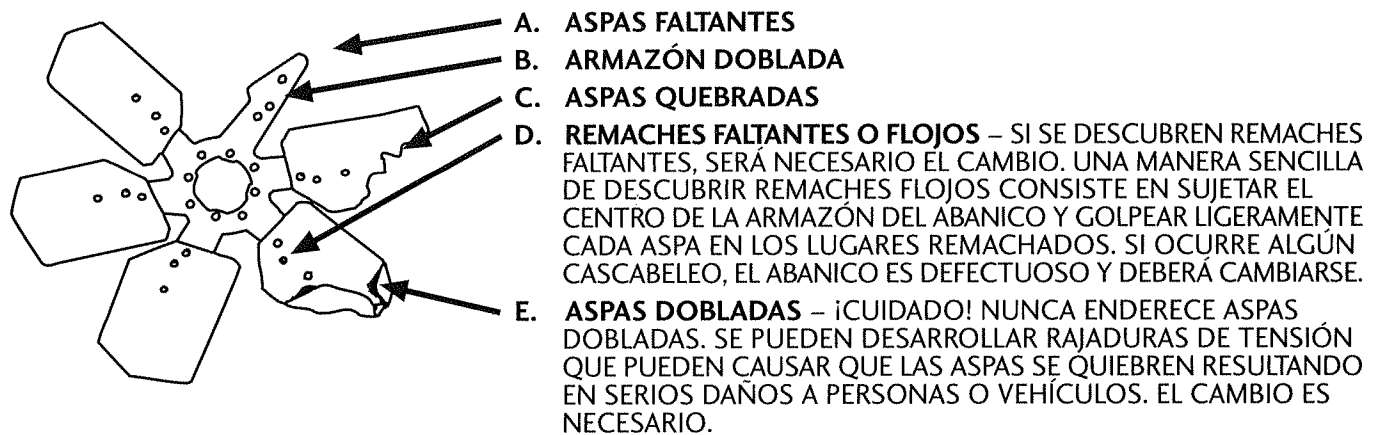
FIG. #1 IMPORTANTE: CAMBIE SIEMPRE LOS ABANICOS DAÑADOS Cosas Que Se Deben Observar Al Inspeccionar El Abanico Del Embrague:
